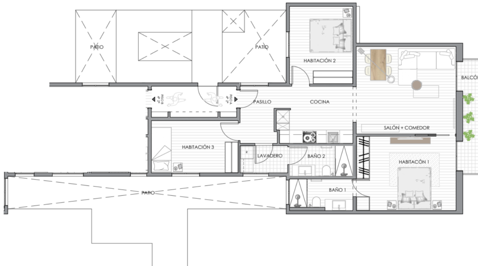
PLANTA VIVIENDA A Esc 1:100
